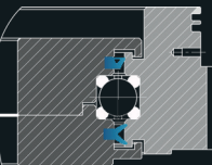
혼합 씰링
